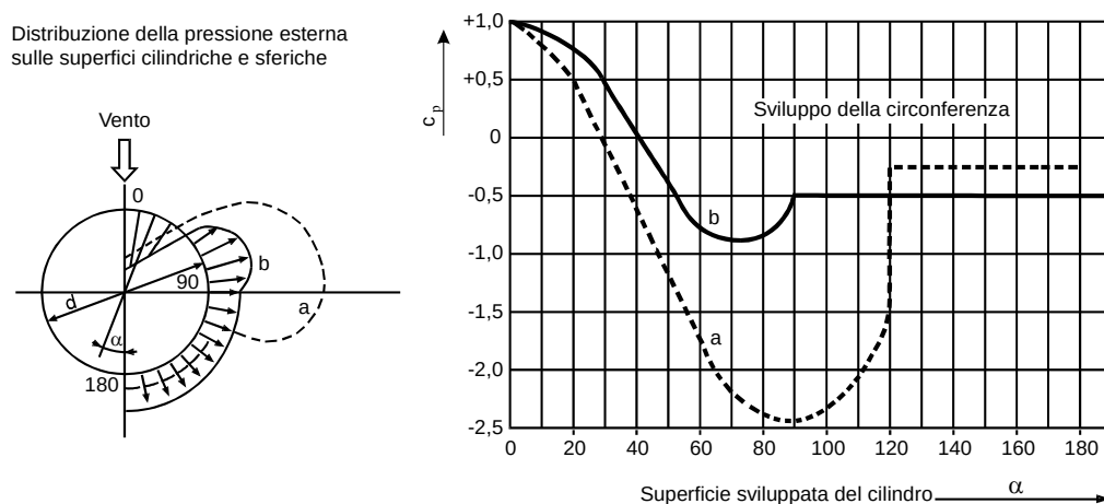
Figura 3.3.12 - Coefficienti di pressione esterna delle superfici cilindriche e sferiche: curva (a) per superfici lisce (metallic, intonaco liscio); curva (b) per superfici ruvide (muratura con giunti di malta, intonaco rustico)
